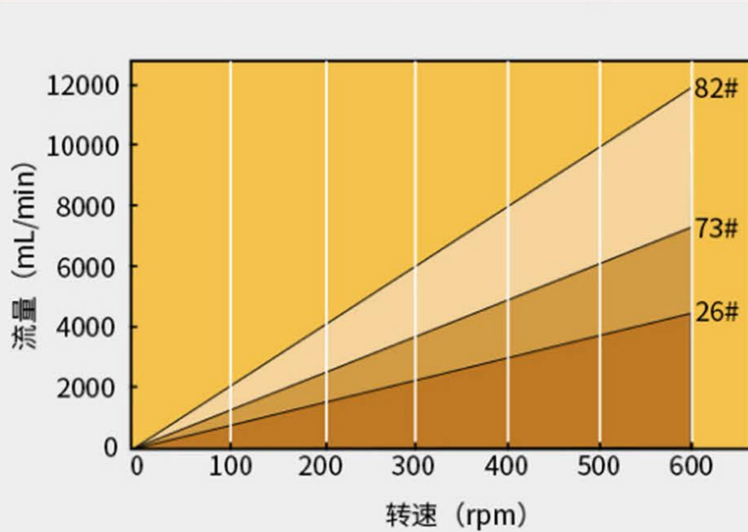
YZ35泵头流量范围 (0.1-600rpm)
