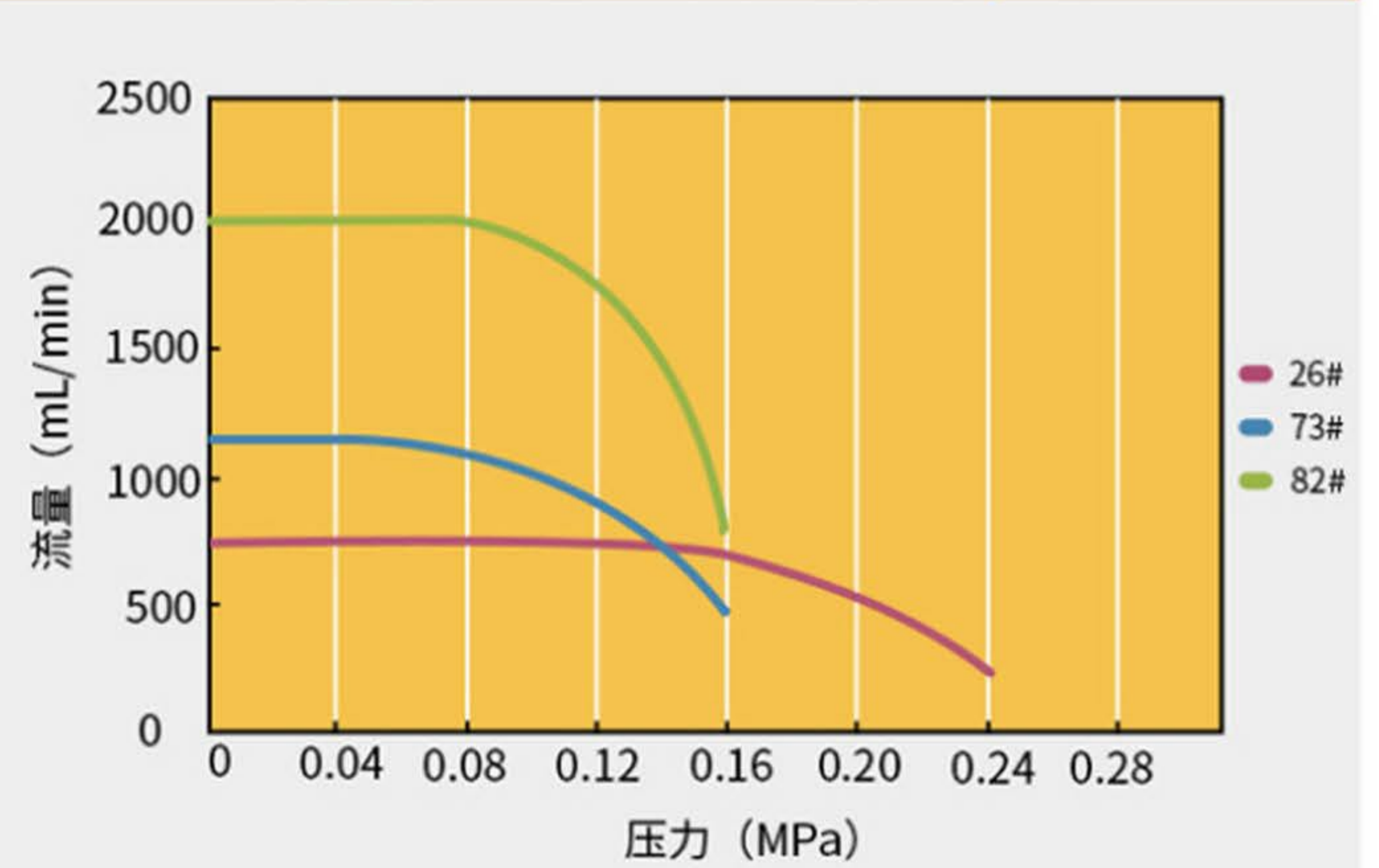
YZ35泵头压力曲线图 (100rpm)
