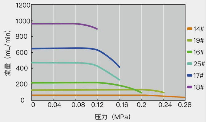
DY15泵头压力/流量曲线图 (100rpm)
